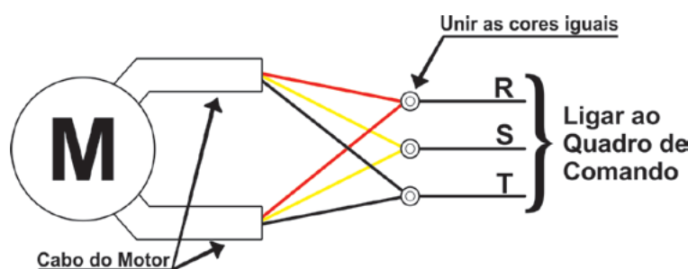
Motor com dois cabos (tensão fixa)
